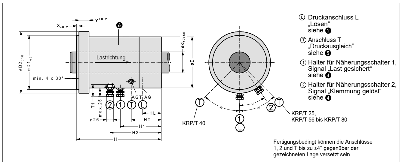
Abb. 1: Abmessungen Absturzsicherung KRP/T (Download von CAD-Daten aus dem Internet: www.sitema.de)
