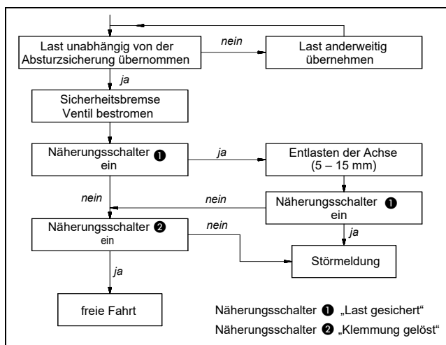
Abb. 6: Klemmung lösen
