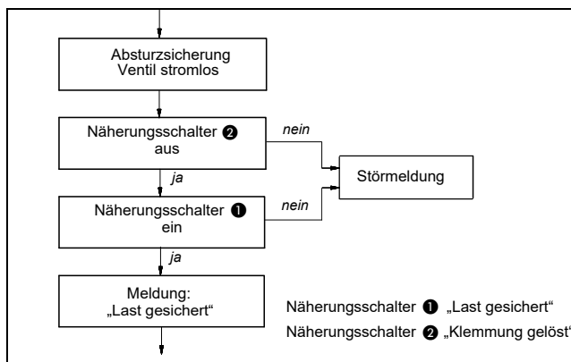
Abb. 5: Last sichern
